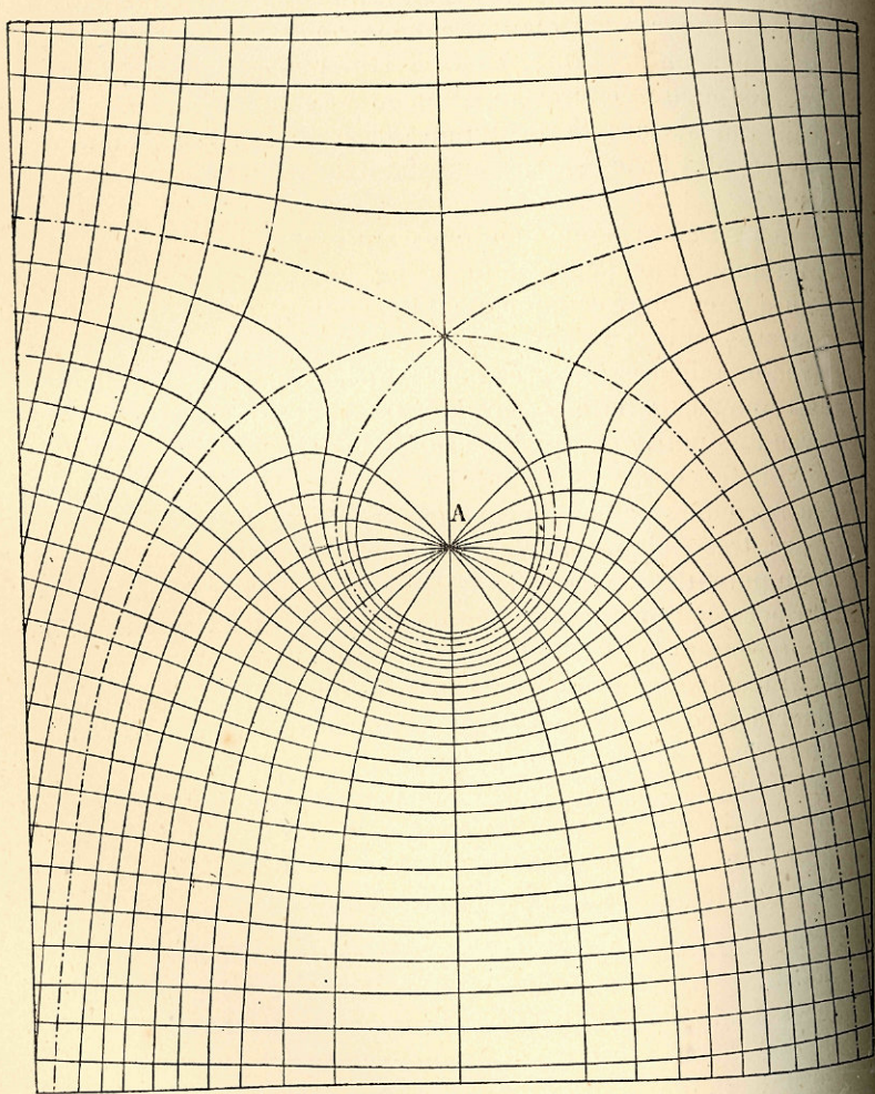
Lignes de force et surfaces équipotentiellles.
