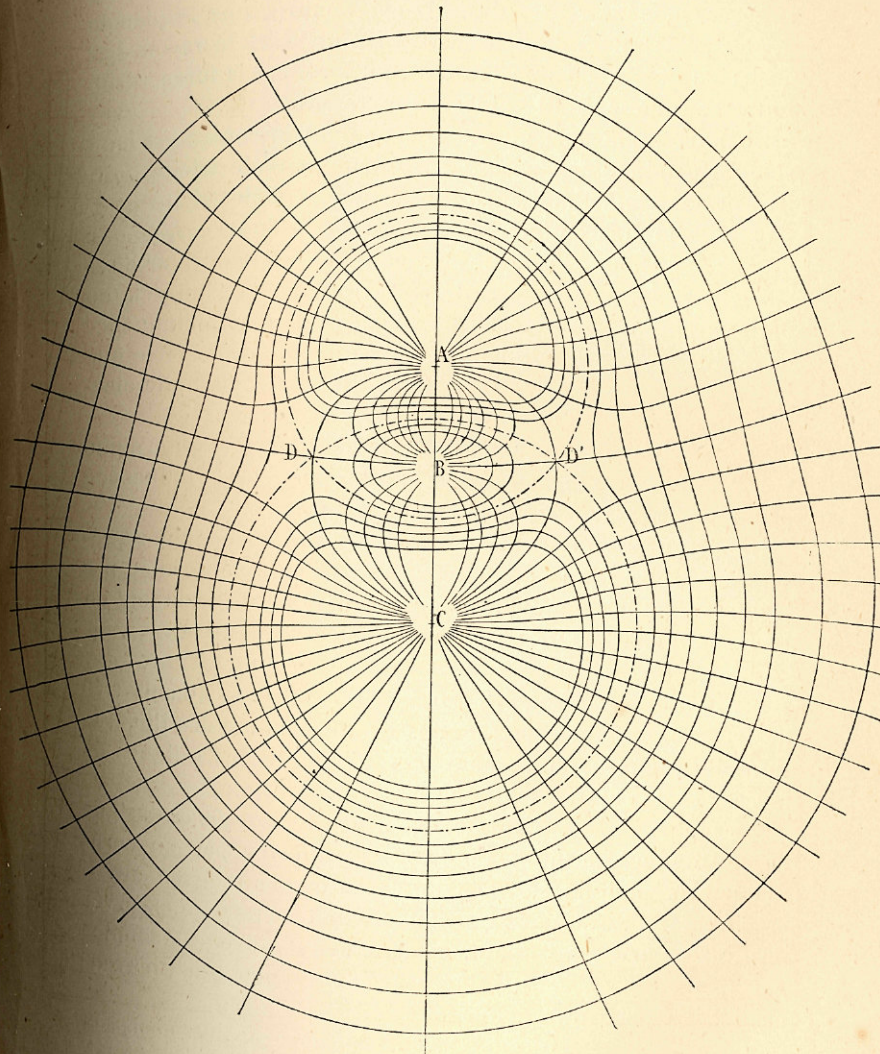
Lignes de force et surfaces équipotentiellles.
