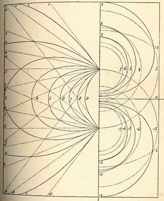
Surfaces équipotentielles.
